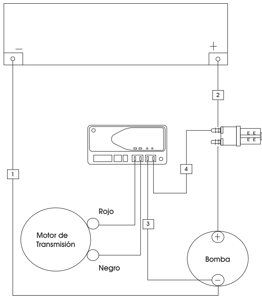
DIAGRAMA DEL CABLEADO (UTILIZADO HASTA EL NO. DE SERIE 7311905397)
