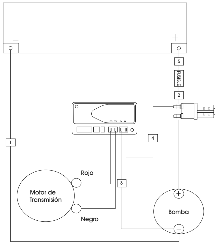
DIAGRAMA DEL CABLEADO (UTILIZADO HASTA EL NO. DE SERIE 7311905398)
