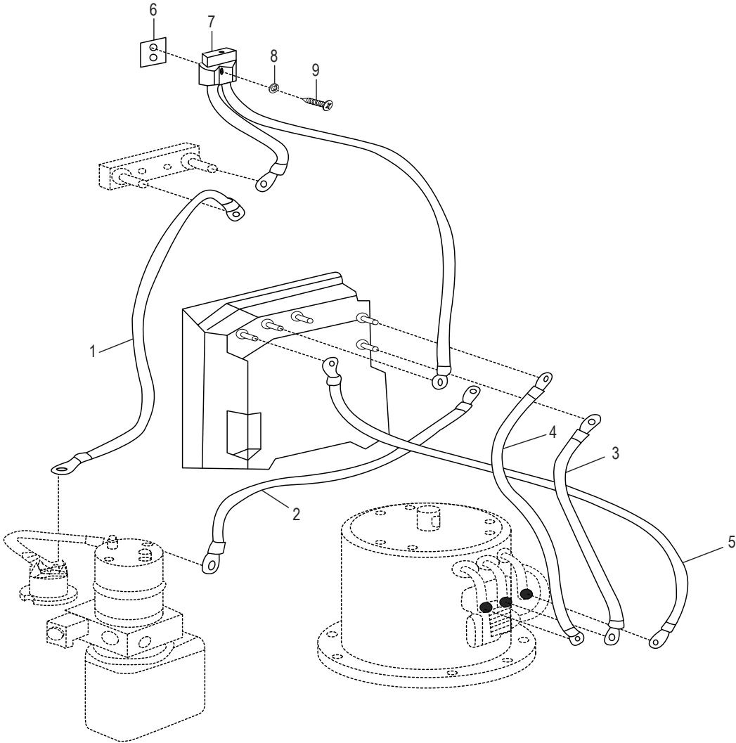
LISTA DE PARTES DEL CABLEADO
