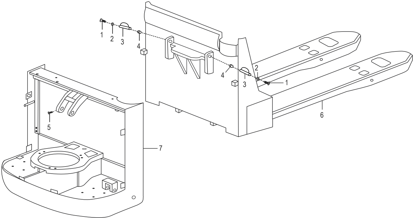
DIAGRAMA DEL ARMAZÓN
