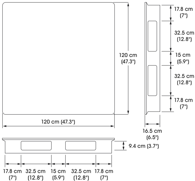
VISTA SUPERIOR
