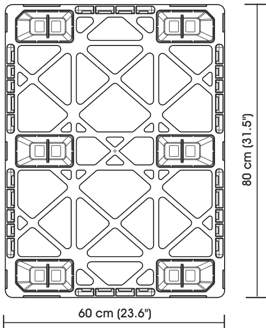
VISTA SUPERIOR
