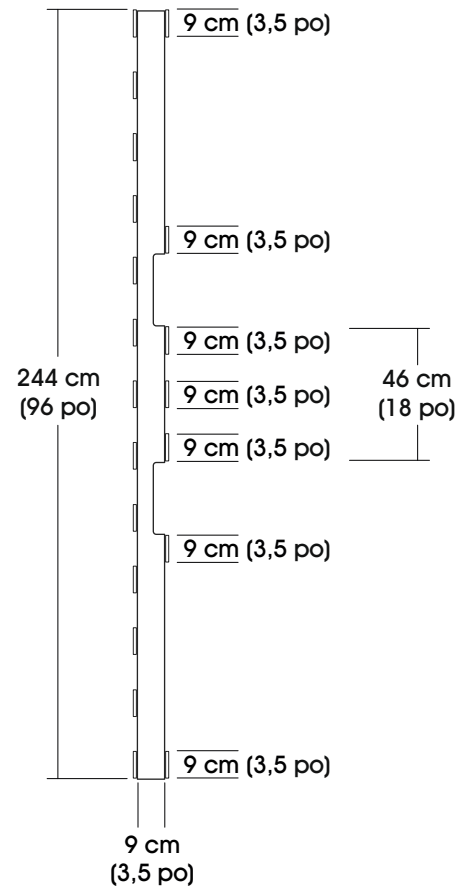
VUE LATÉRALE
