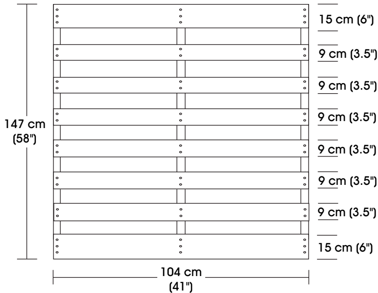
VISTA SUPERIOR
