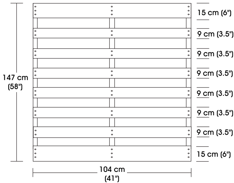
VISTA SUPERIOR
