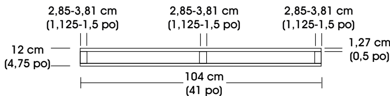
VUE LATÉRALE
