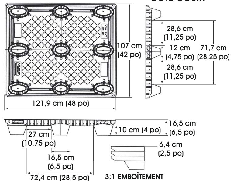
VUE DU CÔTÉ COURT
