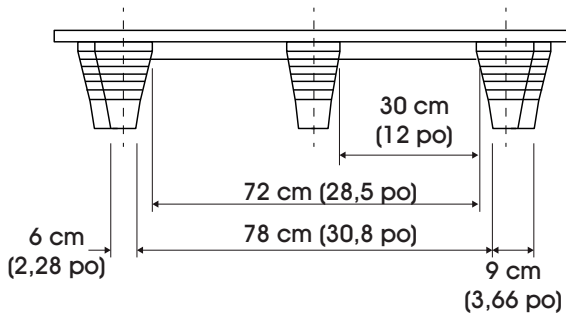
VUE LATÉRALE
